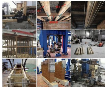
学生参与古建筑修复加固科研试验
